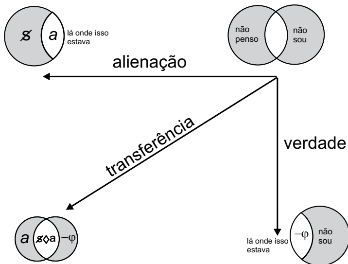
Figura 5: Primeiro semi-grupo: a transferência e o vértice do impasse
