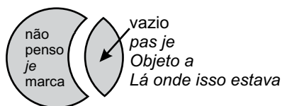
Figura 3: Conjuntos do vértice esquerdo
