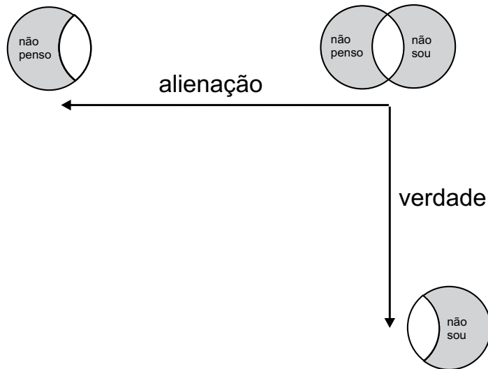
Figura 1: Ponto de partida e primeiras operações
