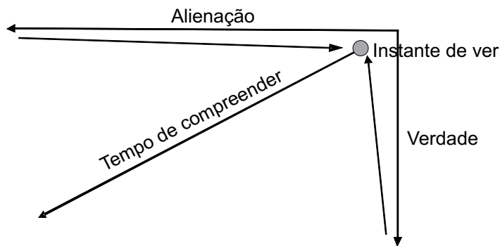
Figura 6: Os tempos lógicos no primeiro semi-grupo
